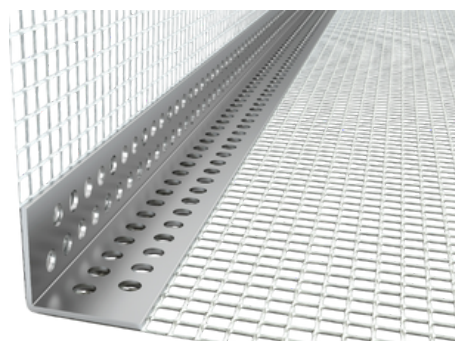
Paraspigolo in alluminio con rete 8x12
