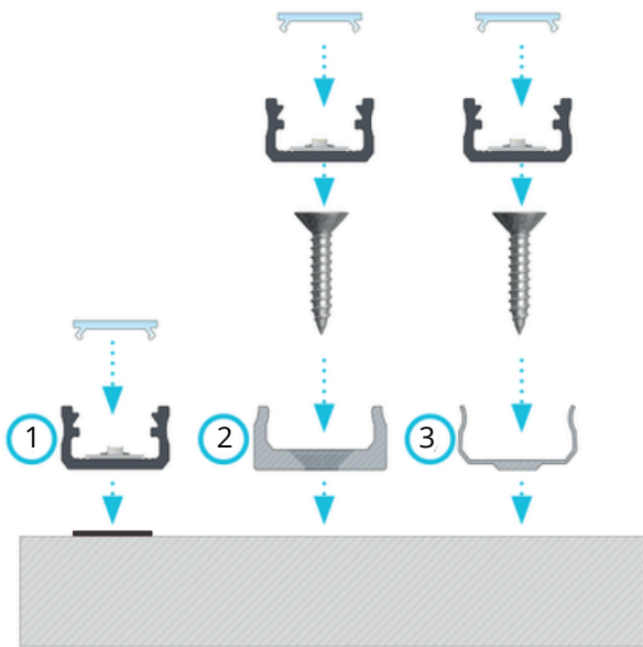
Istruzioni di montaggio del profilo "Lumo" con cover, (1) con nastro biadesivo, (2) con basetta di fissaggio "Lumo" MINI, (3) con basetta di fissaggio in metallo "Lumo".
