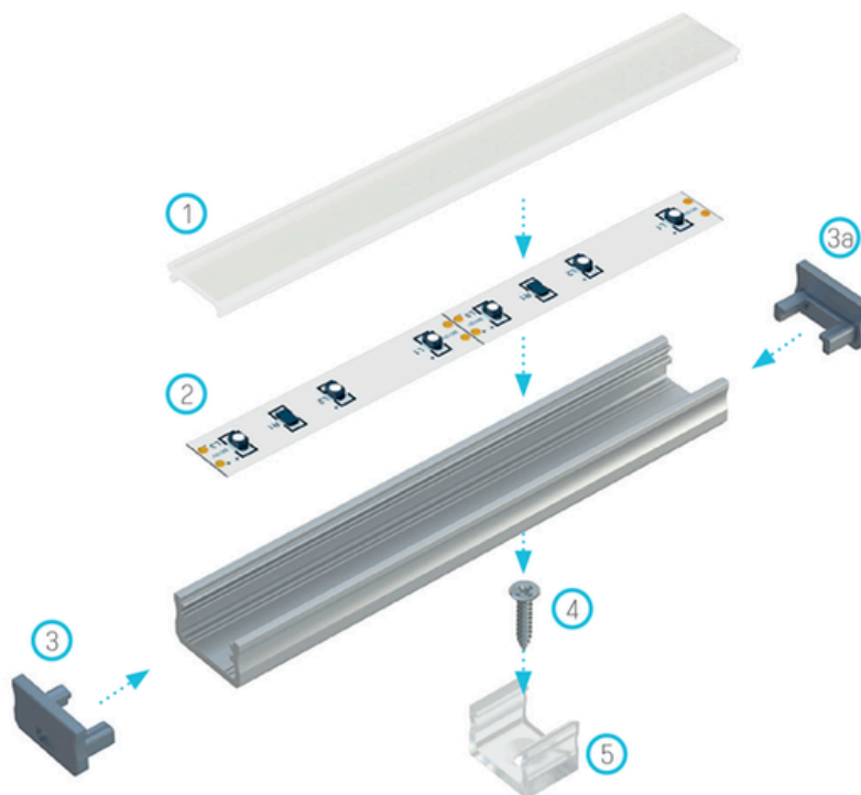
Schema di montaggio degli elementi del sistema di illuminazione con l'uso del profilo "Lumo" e (1) della cover, (2) della striscia LED, (3) del tappo con foro, (3a) del tappo senza foro, (4) della vite di montaggio, (5) della basetta di fissaggio "Lumo" MINI.
