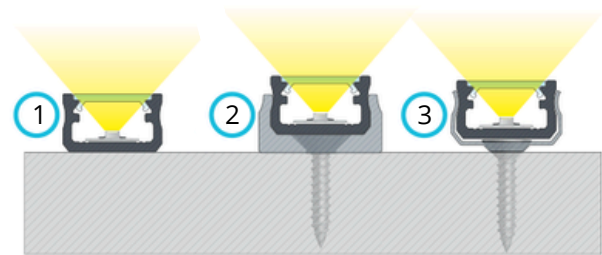
Effetto finale del montaggio del profilo "Lumo" con cover, (1) con nastro biadesivo, (2) con basetta di fissaggio "Lumo" MINI, (3) con basetta di fissaggio in metallo "Lumo".
