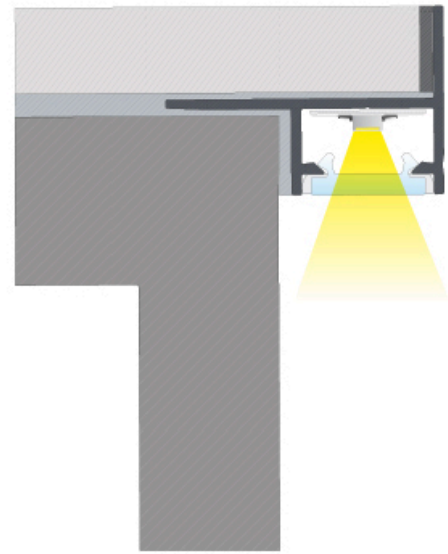
Effetto finale del montaggio per il profilo "Mino" con copertura "Forte".
