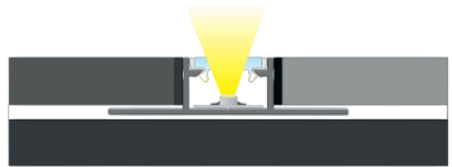
Effetto finale del montaggio per il profilo "Vira" con copertura "Forte".
